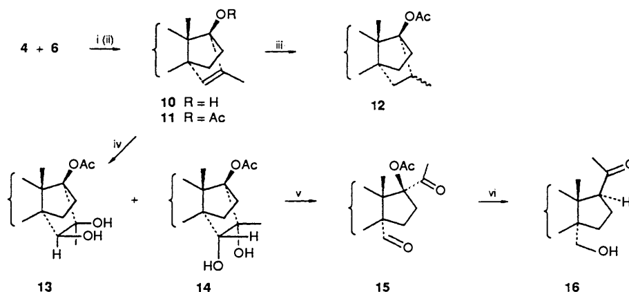
Scheme 2 Reagents and conditions: i, \text{Na}-\text{Hg} , \text{Na}_2\text{HPO}_4 , 0-25^\circ\text{C} ; ii, \text{Ac}_2\text{O}-p\text{TsOH} , 0^\circ\text{C} ; iii, \text{Pd}-\text{C} , \text{H}_2 ; iv, \text{OsO}_4-\text{C}_5\text{H}_5\text{N} , 25^\circ\text{C} ; v, \text{NaIO}_4 , 25^\circ\text{C} ; vi, \text{Ca}-\text{NH}_3 , -78^\circ\text{C}
